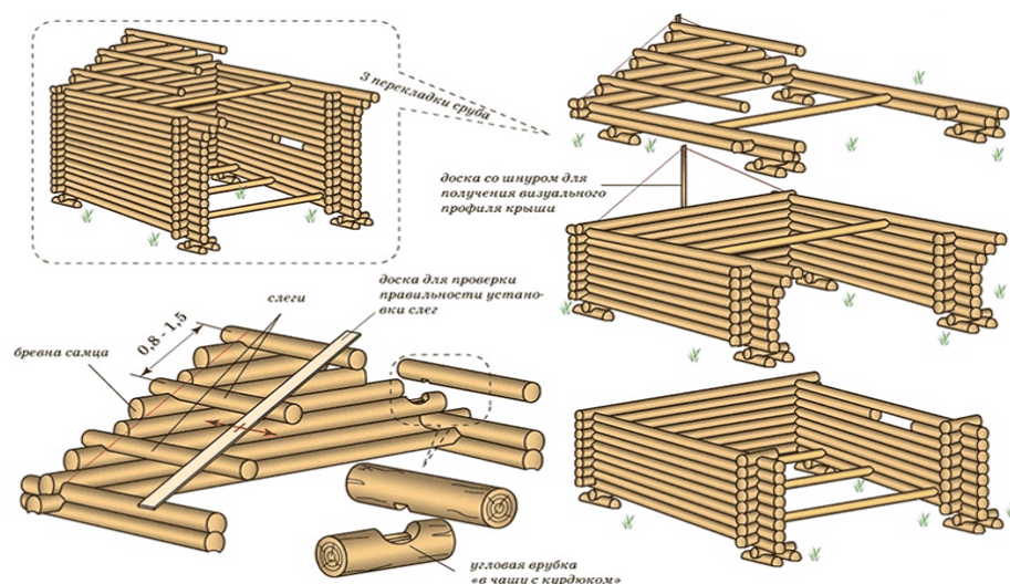
Схема возведения «самцовой» крыши
